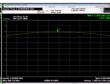
2440MHz
