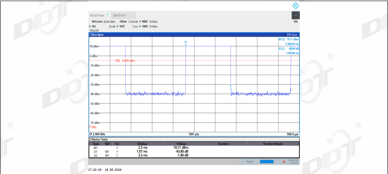
SRD_2M_Right side_2404
