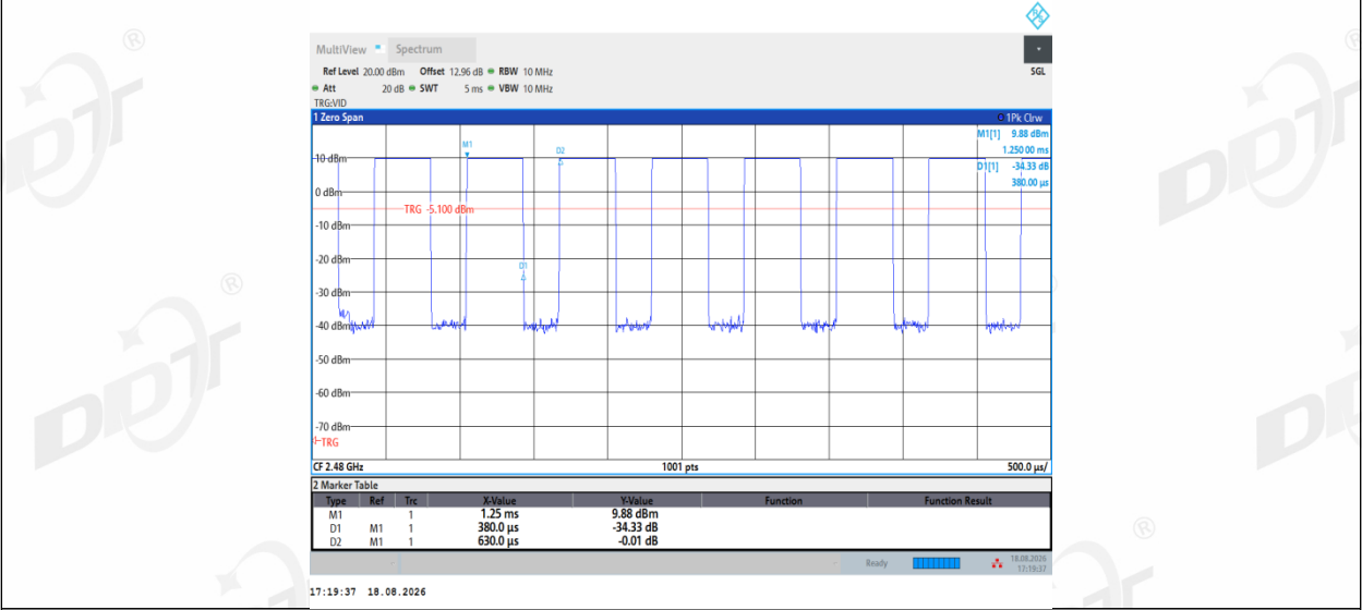
SRD_1M_Right side_2480
