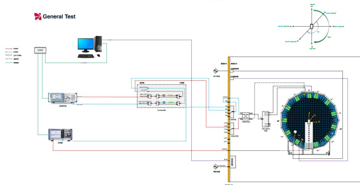
深圳禾邦 RZ1800系统链路图
