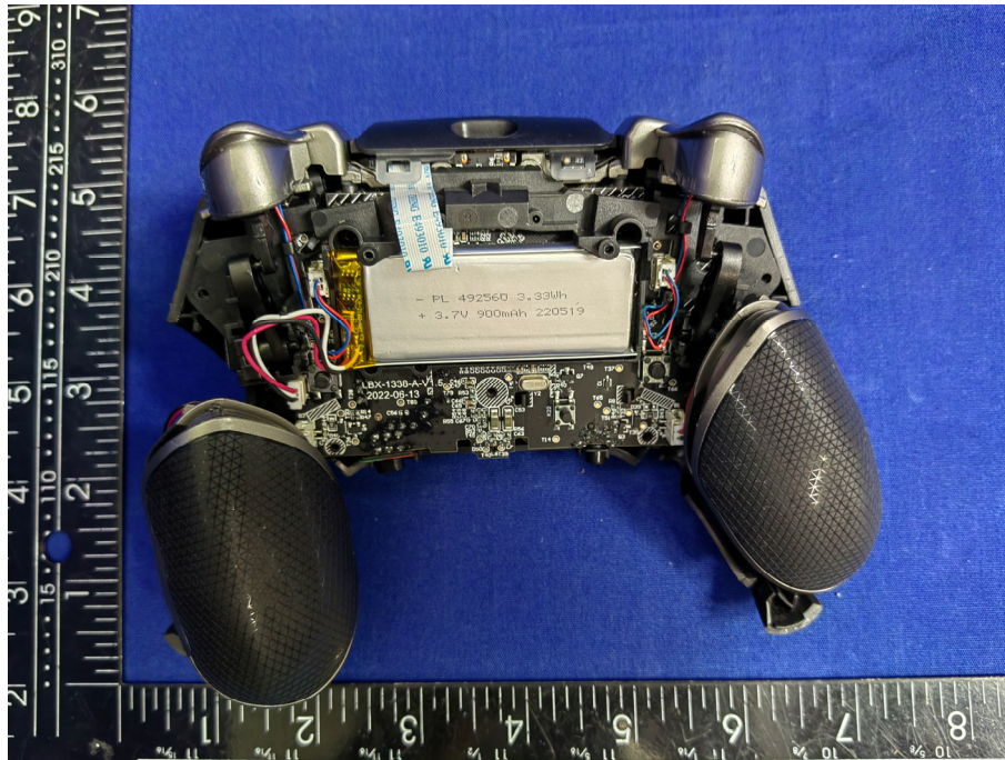
PCB ant
