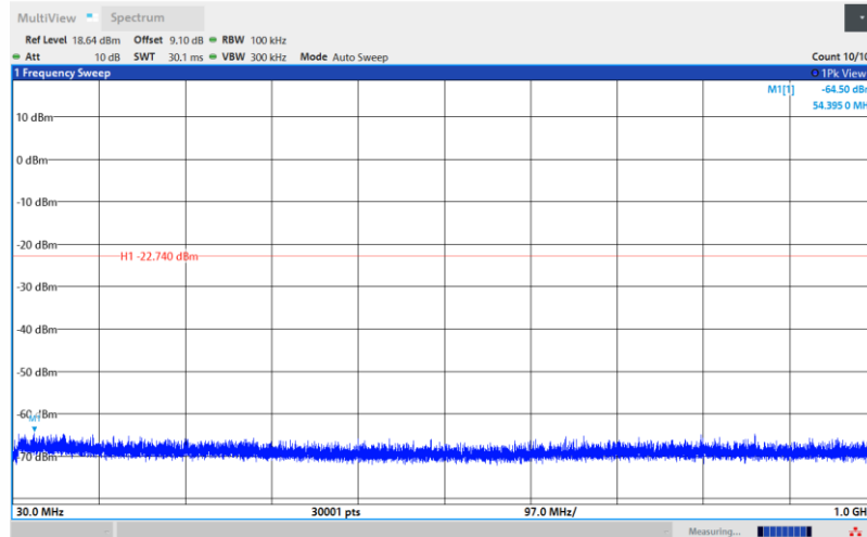
BLE_2M-Ant1-2478-30~1000-PASS
