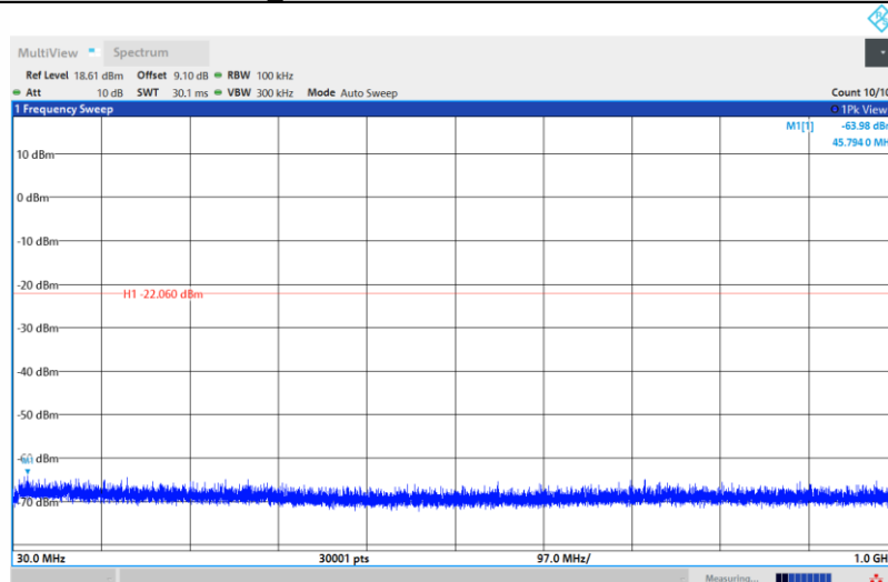
BLE_2M-Ant1-2404-30~1000-PASS
