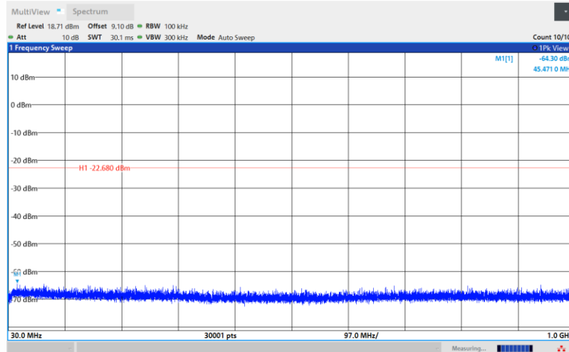
BLE_2M-Ant1-2440-30~1000-PASS
