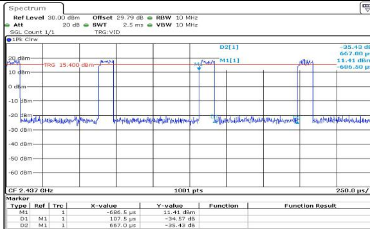
11G-CDD_Ant1_2437
