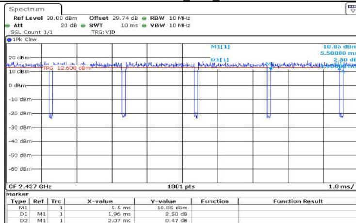
11N20MIMO_Ant1_2437
