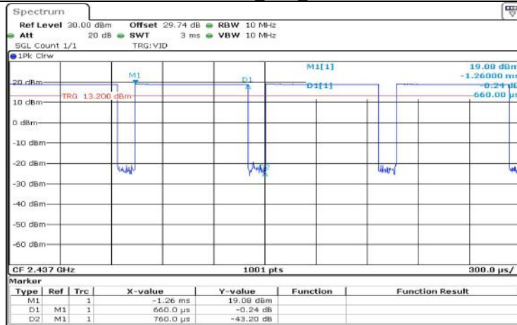
11B-CDD_Ant1_2437
