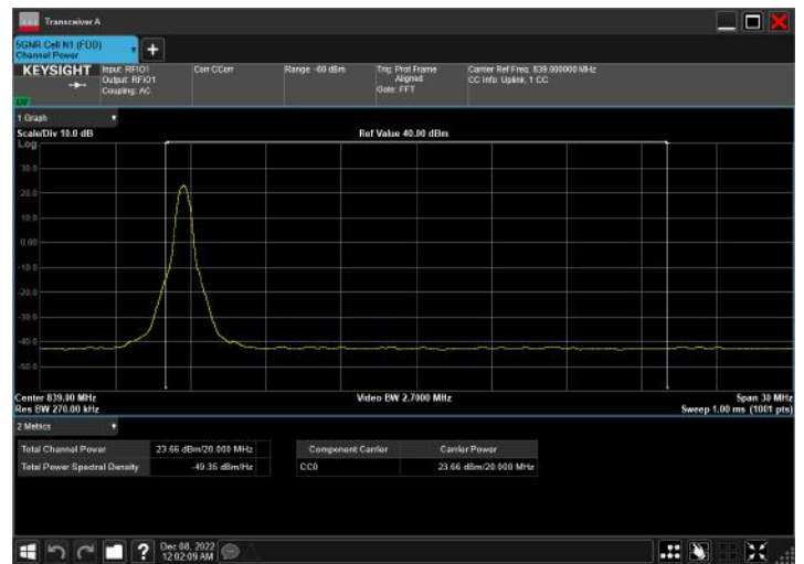
n5_20MHz_15kHz_839MHz_CP-OFDM QPSK_RB1@1
