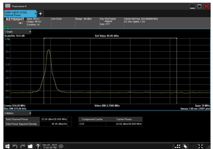
n5_20MHz_15kHz_834MHz_CP-OFDM QPSK_RB1@1
