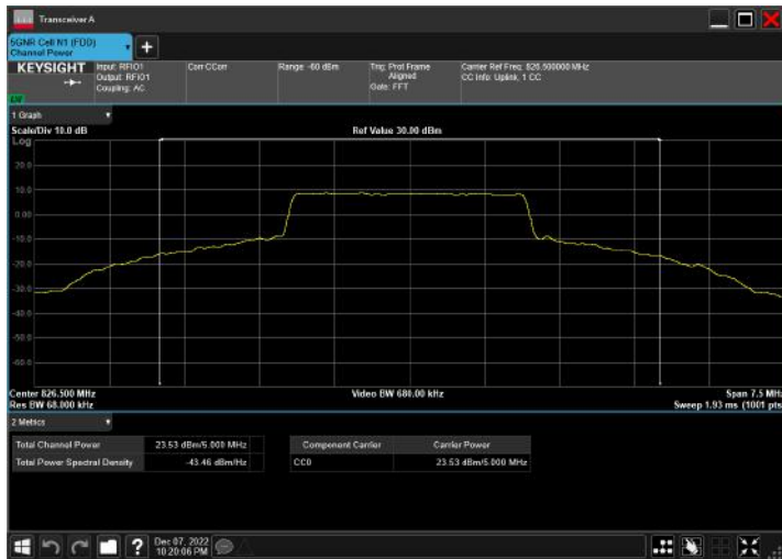
n5_5MHz_15kHz_826.5MHz_CP-OFDM QPSK_RB25@0
