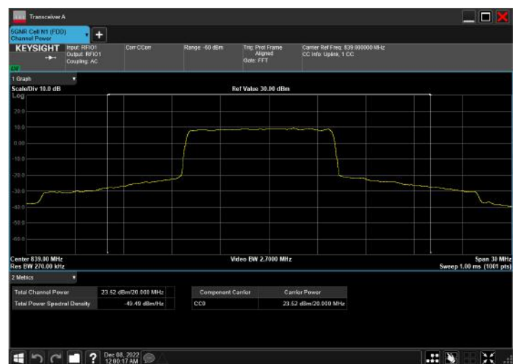
n5_20MHz_15kHz_839MHz_DFT-s-OFDM QPSK_RB50@25
