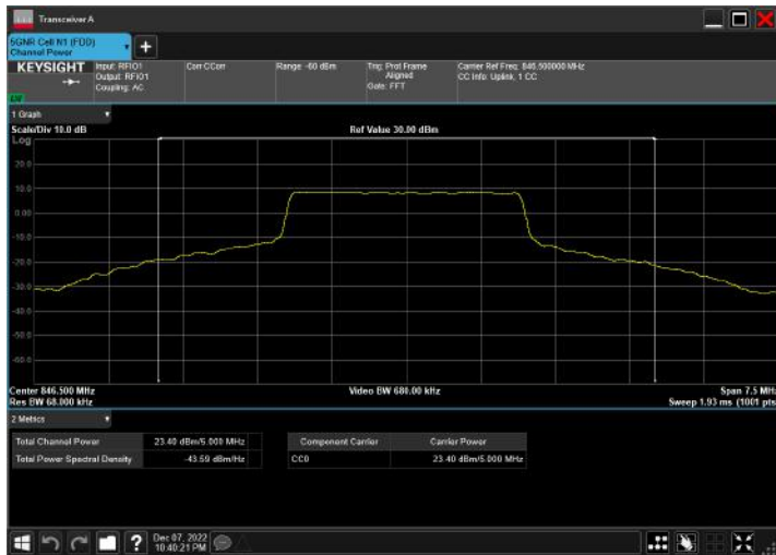
n5_5MHz_15kHz_846.5MHz_CP-OFDM QPSK_RB25@0
