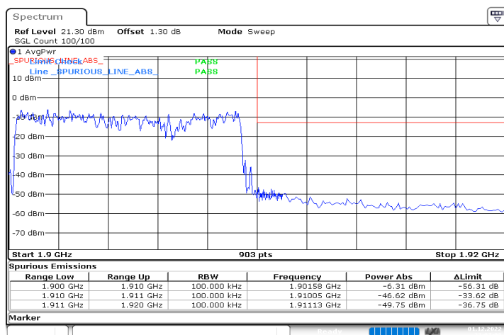
DC_5A_n2A_10MHz|10MHz_15kHz_836.5MHz|1905MHz_DF T-s-OFDM QPSK_RB0|RB50@0
