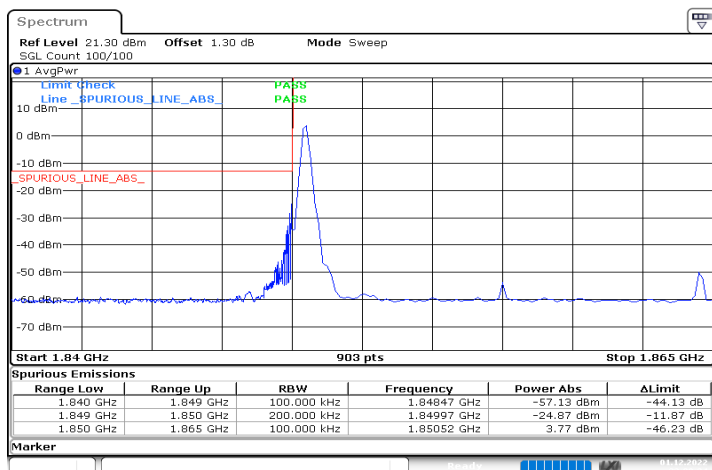
DC_5A_n2A_10MHz|15MHz_15kHz_836.5MHz|1857.5MHz_ DFT-s-OFDM QPSK_RB0|RB1@0
