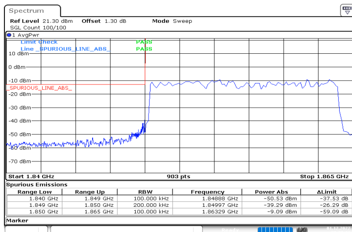
DC_5A_n2A_10MHz|15MHz_15kHz_836.5MHz|1857.5MHz_ DFT-s-OFDM QPSK_RB0|RB75@0
