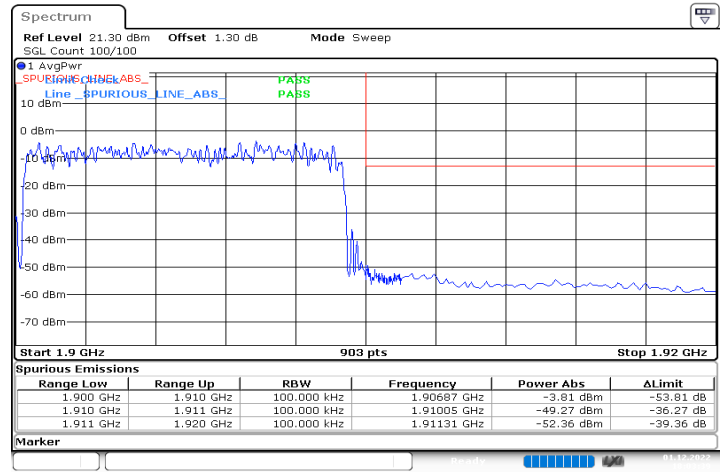
DC_66A_n2A_10MHz|10MHz_15kHz_1745MHz|1905MHz_D FT-s-OFDM QPSK_RB0|RB50@0
