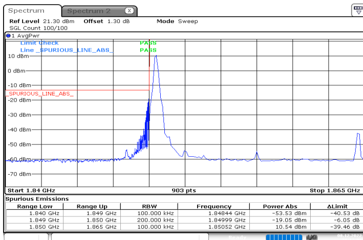
n2_15MHz_15kHz_1857.5MHz_DFT-s-OFDM QPSK_RB1@0
