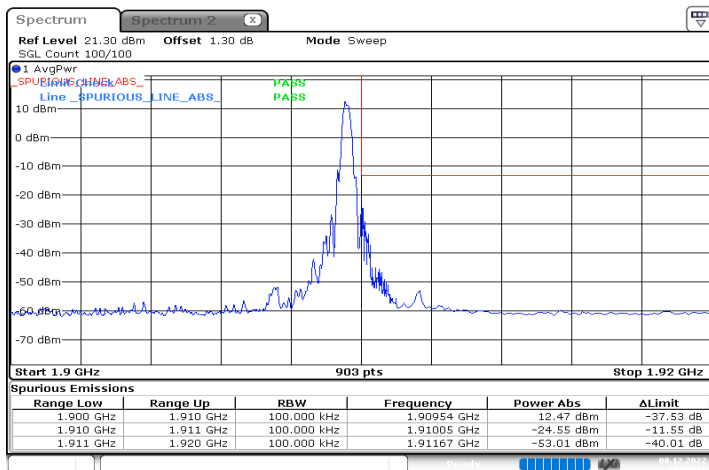
n2_10MHz_15kHz_1905MHz_DFT-s-OFDM QPSK_RB1@51
