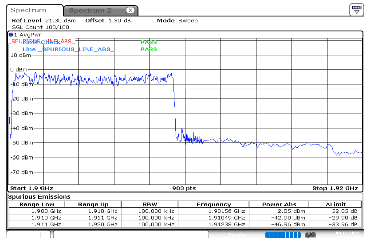
n2_10MHz_15kHz_1905MHz_DFT-s-OFDM QPSK_RB50@0
