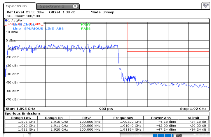
n2_15MHz_15kHz_1902.5MHz_DFT-s-OFDM QPSK_RB75@0
