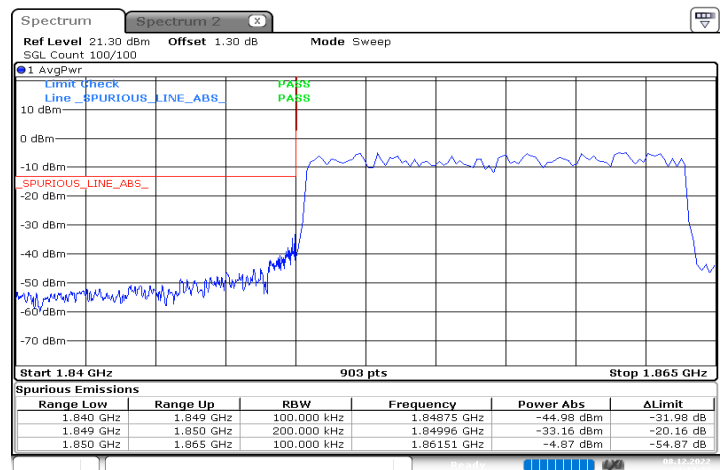
n2_15MHz_15kHz_1857.5MHz_DFT-s-OFDM QPSK_RB75@0
