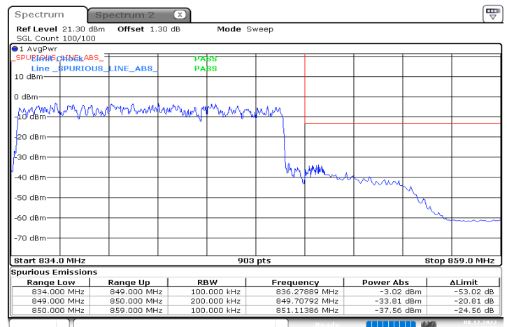
n5_15MHz_15kHz_841.5MHz_DFT-s-OFDM QPSK_RB75@0
