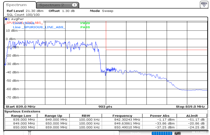
n5_10MHz_15kHz_844MHz_DFT-s-OFDM QPSK_RB50@0
