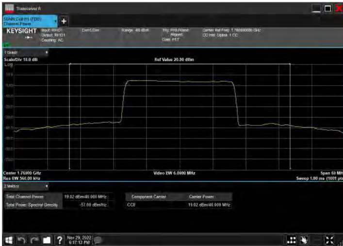
DC_2A_n66A_10MHz|40MHz_15kHz_1905MHz|1760MHz_Q PSK|CP-OFDM QPSK_RB12@38|RB108@54
