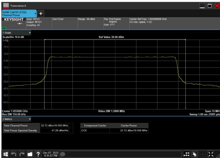
n2_10MHz_15kHz_1855MHz_DFT-s-OFDM 16 QAM_RB50@0
