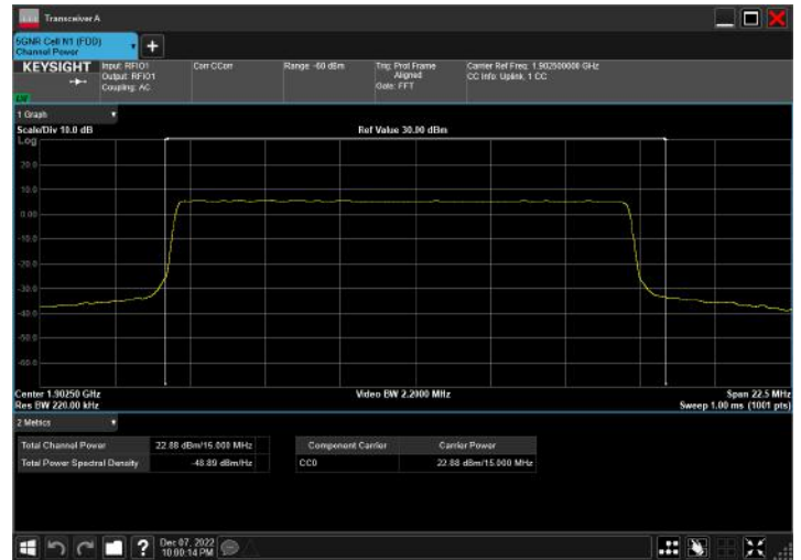
n2_15MHz_15kHz_1902.5MHz_DFT-s-OFDM QPSK_RB75@0
