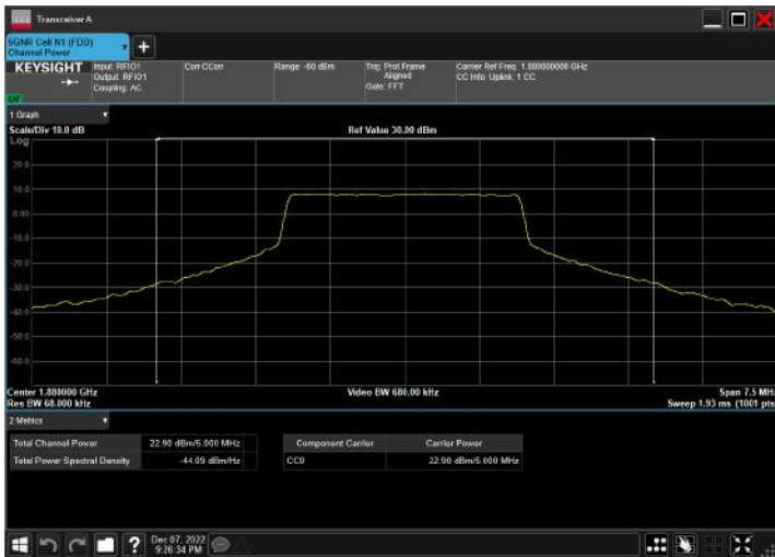
n2_5MHz_15kHz_1880MHz_CP-OFDM QPSK_RB25@0
