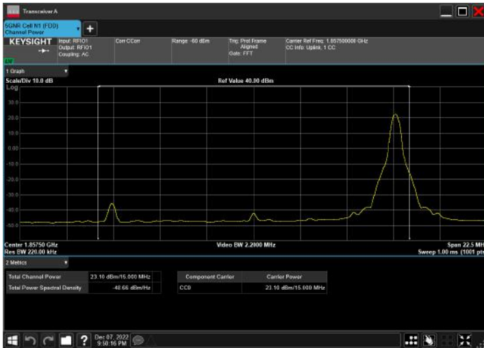
n2_15MHz_15kHz_1857.5MHz_DFT-s-OFDM QPSK_RB1@77
