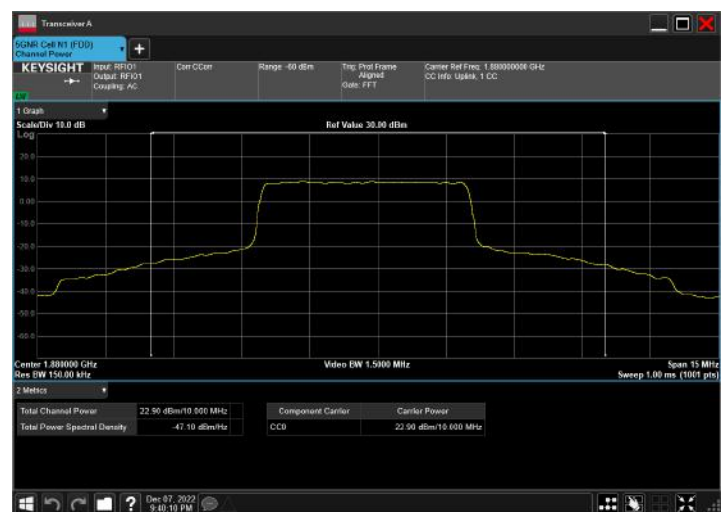
n2_10MHz_15kHz_1880MHz_DFT-s-OFDM QPSK_RB25@12
