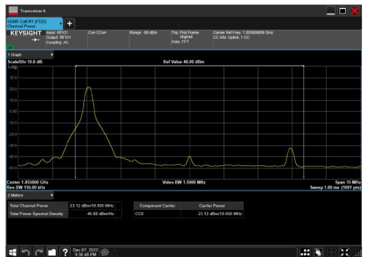
n2_10MHz_15kHz_1855MHz_CP-OFDM QPSK_RB1@1
