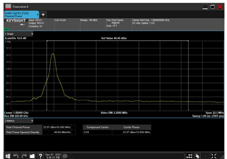
n2_15MHz_15kHz_1880MHz_CP-OFDM QPSK_RB1@1
