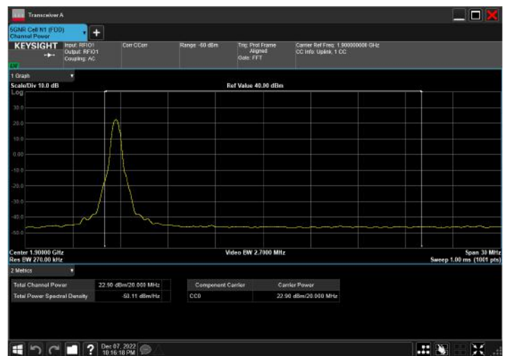
n2_20MHz_15kHz_1900MHz_CP-OFDM QPSK_RB1@1
