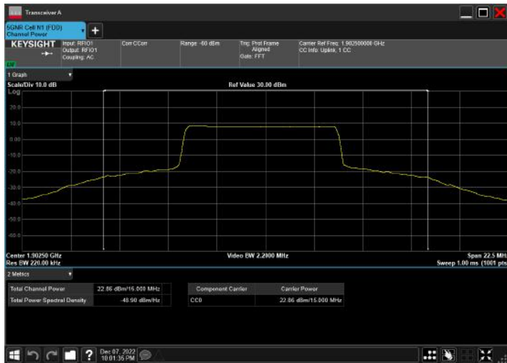
n2_15MHz_15kHz_1902.5MHz_CP-OFDM QPSK_RB79@0
