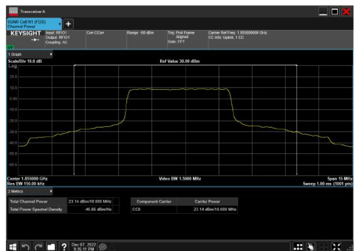
n2_10MHz_15kHz_1855MHz_DFT-s-OFDM QPSK_RB25@12
