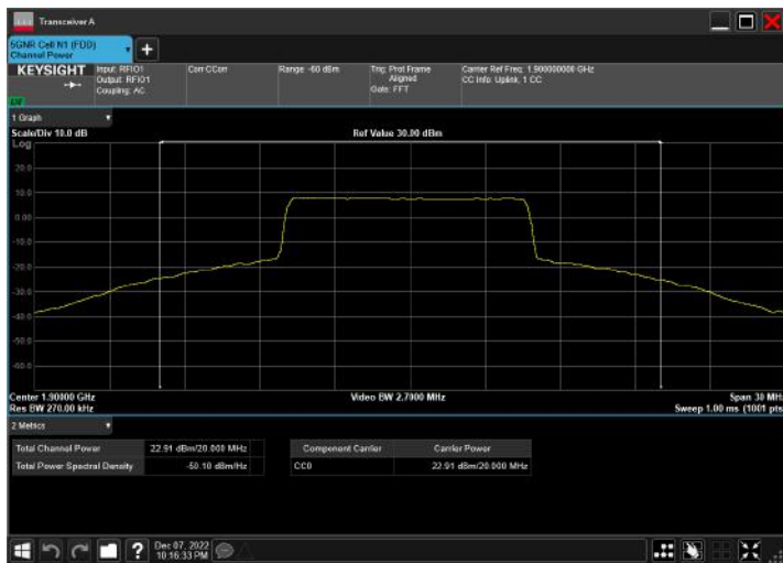
n2_20MHz_15kHz_1900MHz_CP-OFDM QPSK_RB106@0
