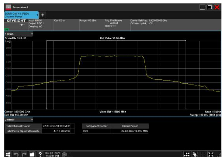
n2_10MHz_15kHz_1905MHz_DFT-s-OFDM QPSK_RB25@12
