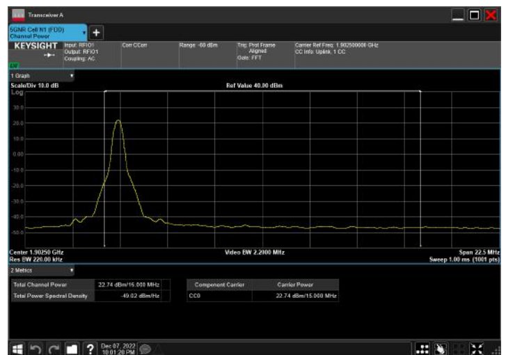
n2_15MHz_15kHz_1902.5MHz_CP-OFDM QPSK_RB1@1
