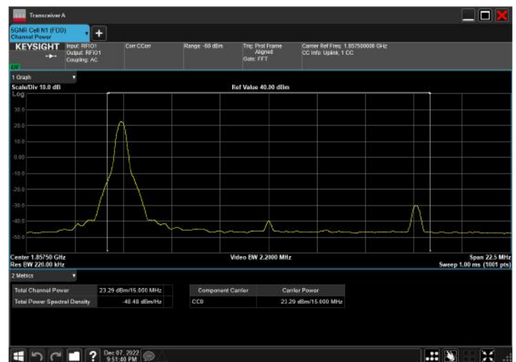
n2_15MHz_15kHz_1857.5MHz_CP-OFDM QPSK_RB1@1
