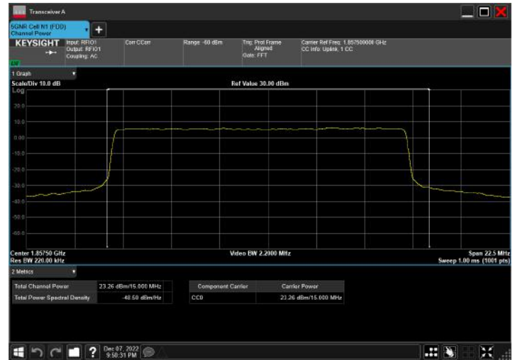
n2_15MHz_15kHz_1857.5MHz_DFT-s-OFDM QPSK_RB75@0
