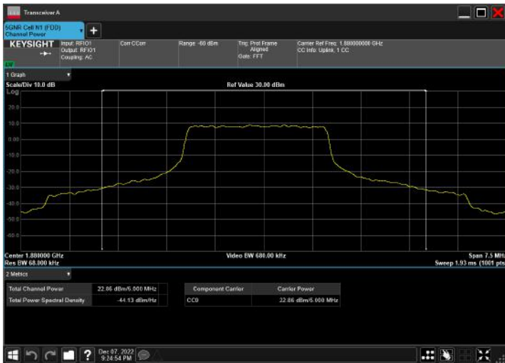
n2_5MHz_15kHz_1880MHz_DFT-s-OFDM QPSK_RB25@0
