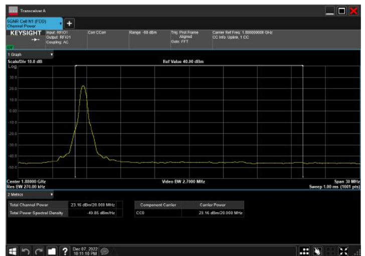
n2_20MHz_15kHz_1880MHz_CP-OFDM QPSK_RB1@1
