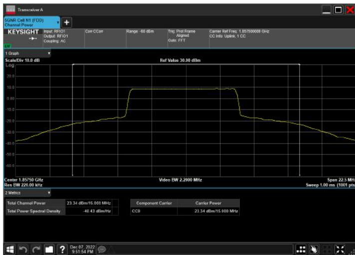
n2_15MHz_15kHz_1857.5MHz_CP-OFDM QPSK_RB79@0
