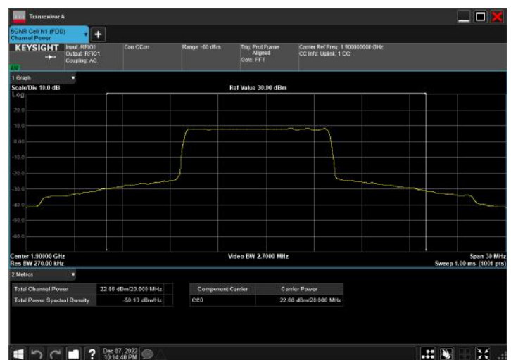
n2_20MHz_15kHz_1900MHz_DFT-s-OFDM QPSK_RB50@25
