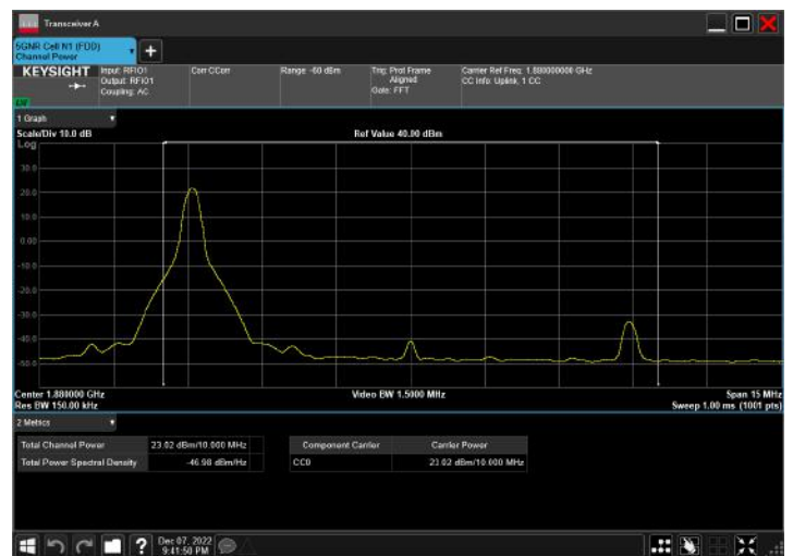
n2_10MHz_15kHz_1880MHz_CP-OFDM QPSK_RB1@1
