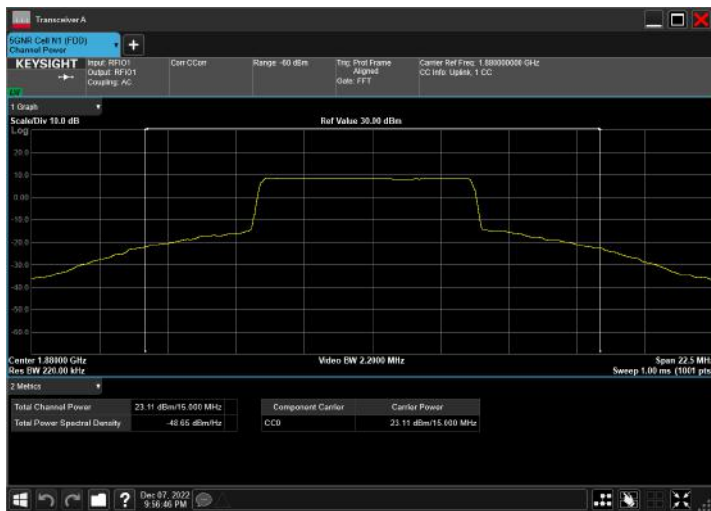
n2_15MHz_15kHz_1880MHz_CP-OFDM QPSK_RB79@0
