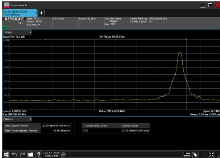
n2_15MHz_15kHz_1902.5MHz_DFT-s-OFDM QPSK_RB1@77
