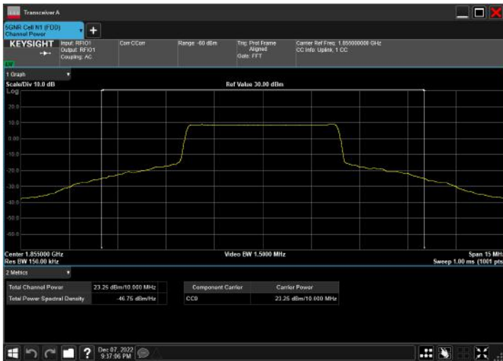
n2_10MHz_15kHz_1855MHz_CP-OFDM QPSK_RB52@0
