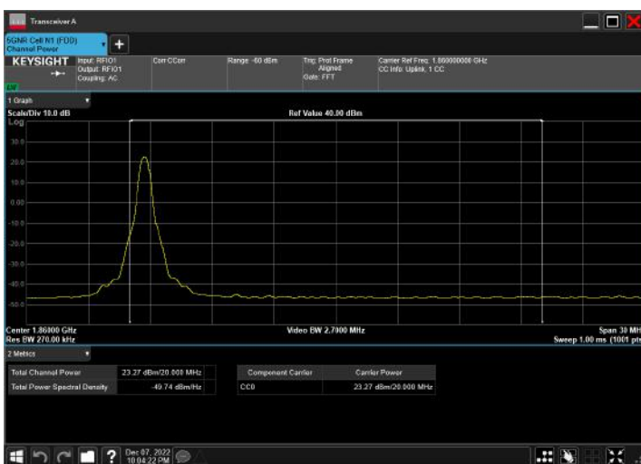
n2_20MHz_15kHz_1860MHz_DFT-s-OFDM QPSK_RB1@1
