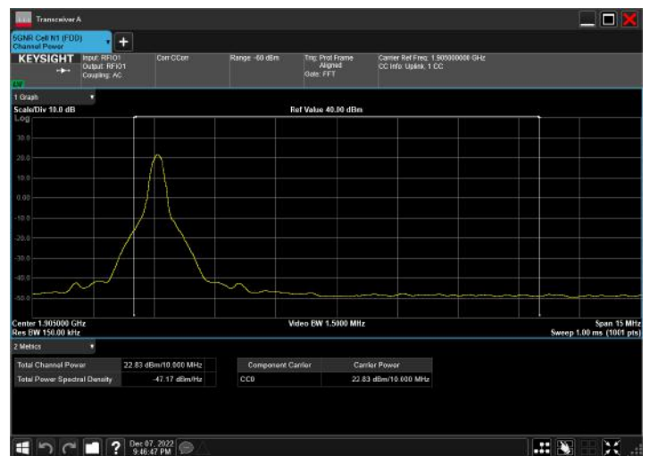
n2_10MHz_15kHz_1905MHz_CP-OFDM QPSK_RB1@1
