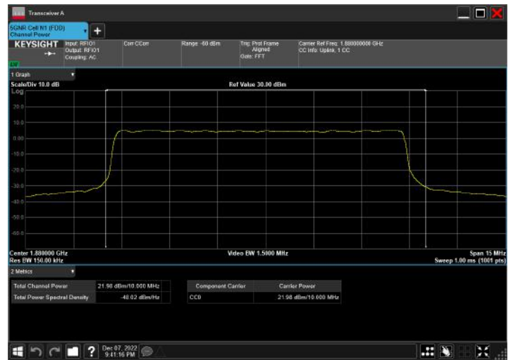
n2_10MHz_15kHz_1880MHz_DFT-s-OFDM 64 QAM_RB50@0
