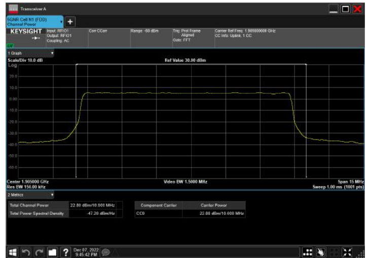
n2_10MHz_15kHz_1905MHz_DFT-s-OFDM 64 QAM_RB50@0
