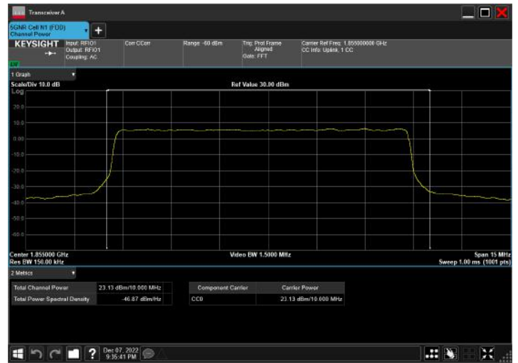
n2_10MHz_15kHz_1855MHz_DFT-s-OFDM 64 QAM_RB50@0
