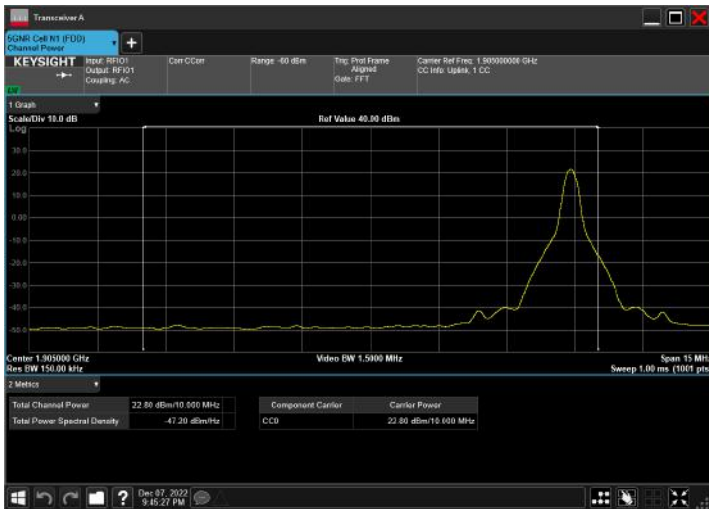
n2_10MHz_15kHz_1905MHz_DFT-s-OFDM 16 QAM_RB50@0
