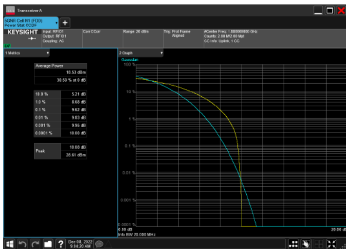
n2_20MHz_15kHz_1880MHz_CP-OFDM QPSK_RB106@0
