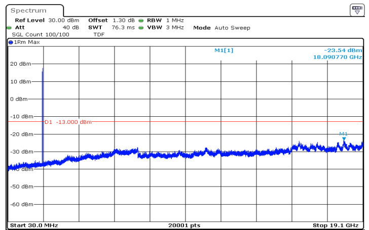
n2_10MHz_15kHz_1880MHz_DFT-s-OFDM QPSK_RB50@0|30MHz_19.1GHz
