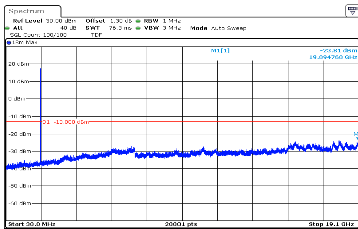
n2_10MHz_15kHz_1905MHz_DFT-s-OFDM QPSK_RB50@0|30MHz_19.1GHz
