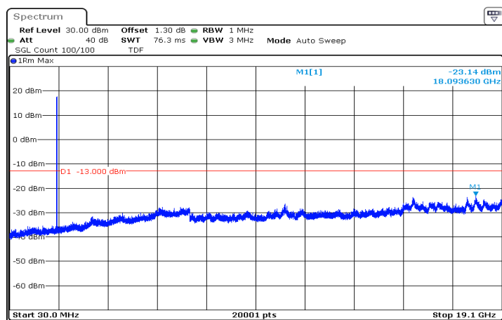
n2_10MHz_15kHz_1855MHz_DFT-s-OFDM QPSK_RB50@0|30MHz_19.1GHz
