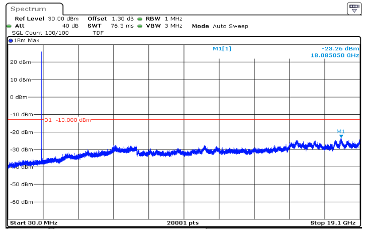
n2_10MHz_15kHz_1855MHz_DFT-s-OFDM QPSK_RB1@0|30MHz_19.1GHz
