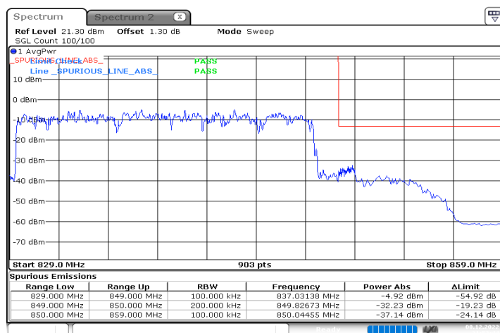
n5_20MHz_15kHz_839MHz_DFT-s-OFDM QPSK_RB100@0
