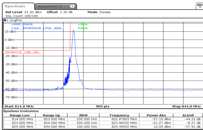
n5_20MHz_15kHz_834MHz_DFT-s-OFDM QPSK_RB1@0
