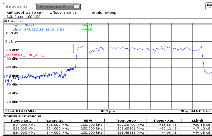
n5_20MHz_15kHz_834MHz_DFT-s-OFDM QPSK_RB100@0
