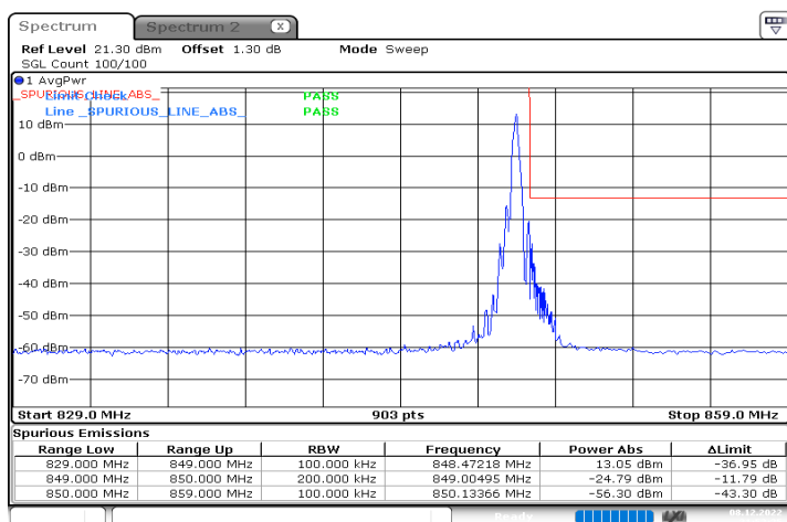
n5_20MHz_15kHz_839MHz_DFT-s-OFDM QPSK_RB1@105
