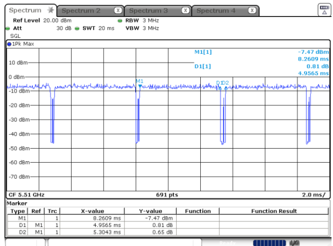
11n (HT40) 5510 MHz
