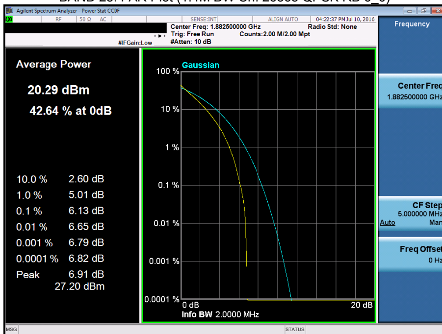
BAND 25. PAR Plot (1.4M BW Ch. 26365 QPSK RB 6_0)
