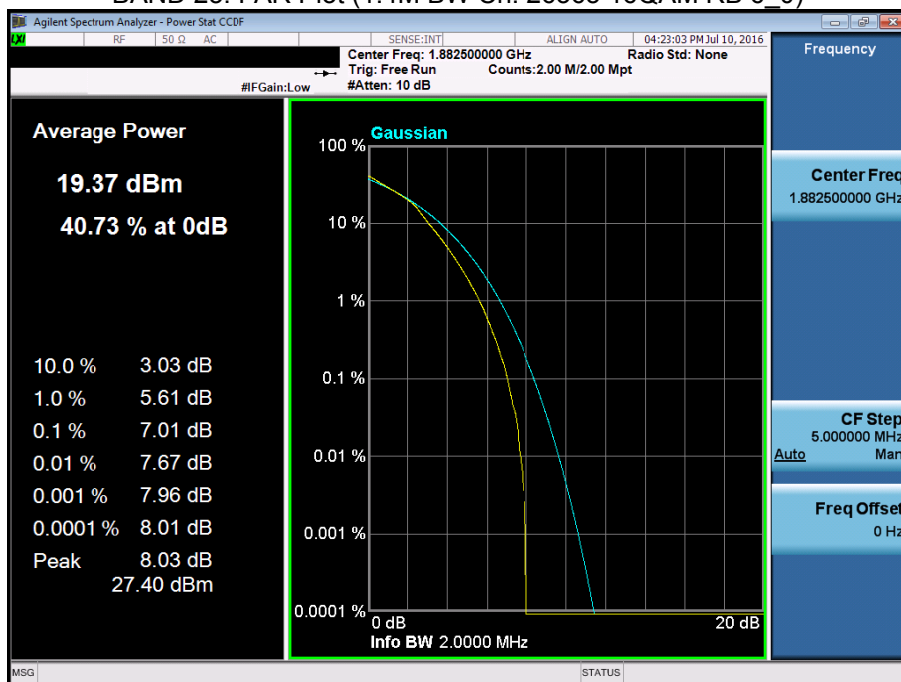
BAND 25. PAR Plot (1.4M BW Ch. 26365 16QAM RB 6_0)
