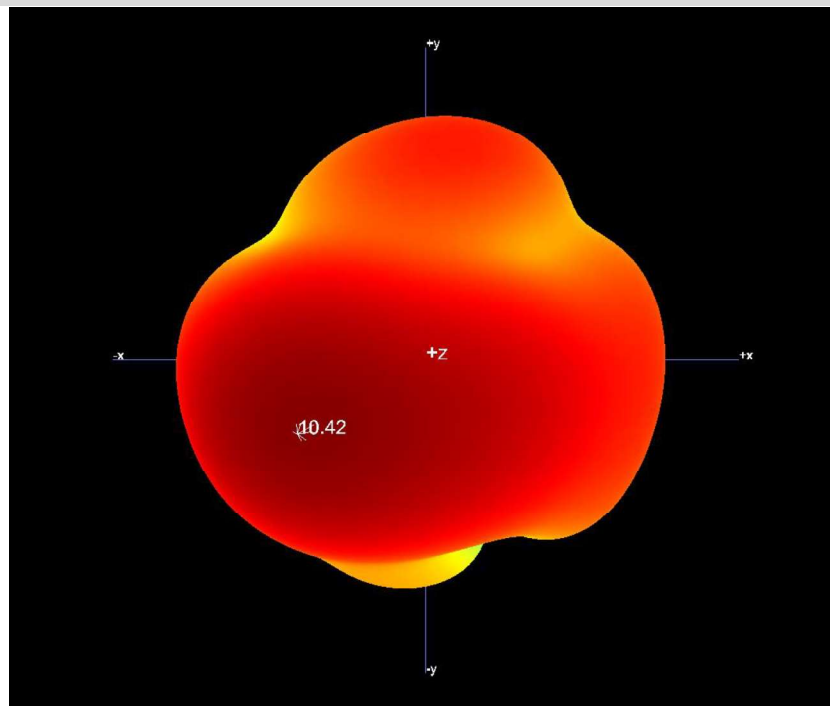
B1.4 3D Pattern for 1710MHz
