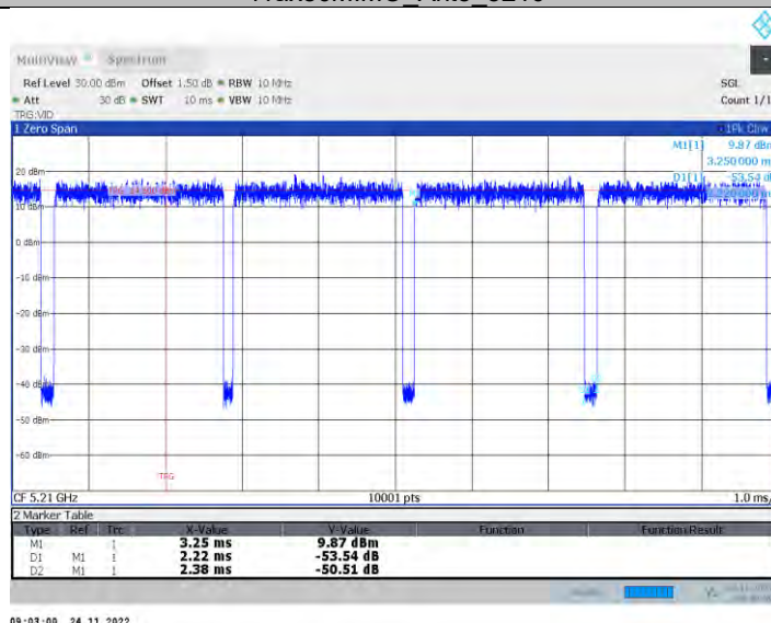
11ax80MIMO Ant6 5210
