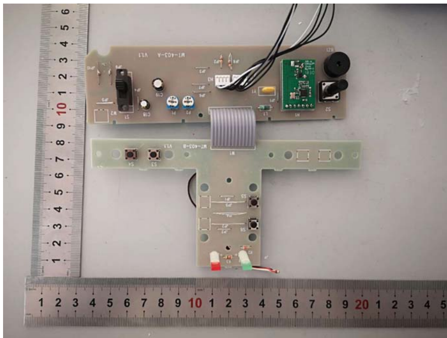
EUT – PCB-1 Bottom Module View
