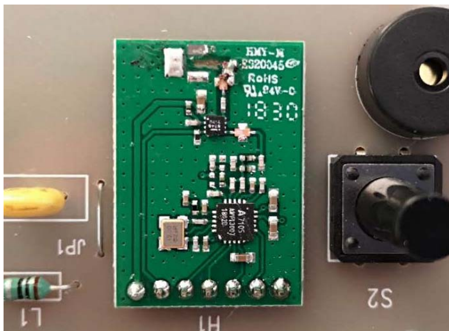
EUT – PCB-1 Bottom Module View
