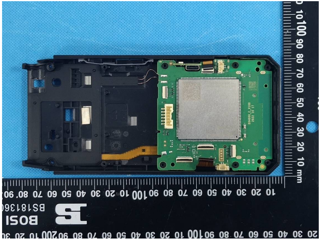
NFC Antenna
