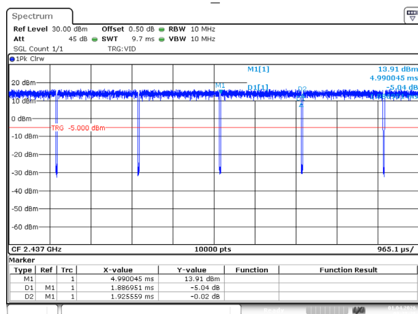
802.11n20_2437MHz
