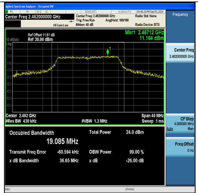
11g-Ant1-2462
