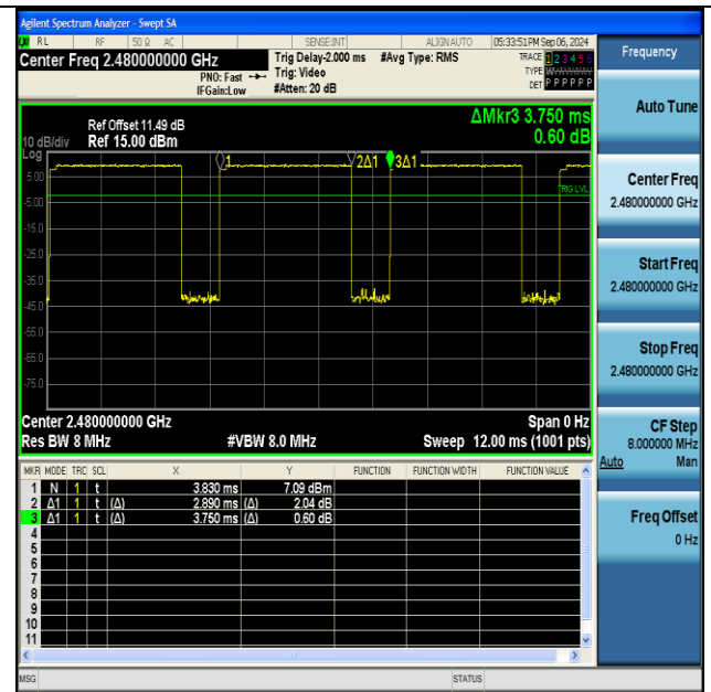
NTNV-2DH5-Ant1-2480
