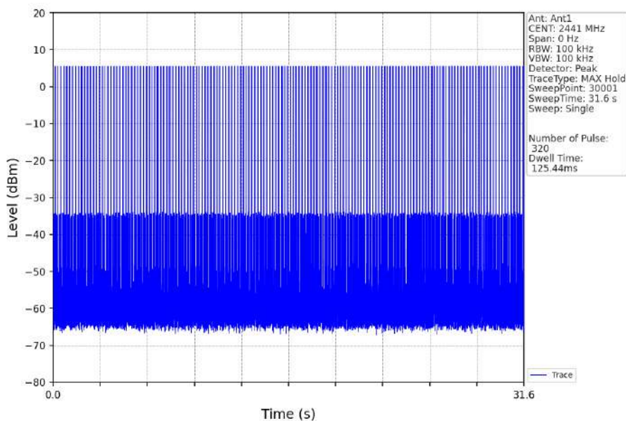
Pi/4DQPSK_2DH1_HOPP_Ant1_NTNV
