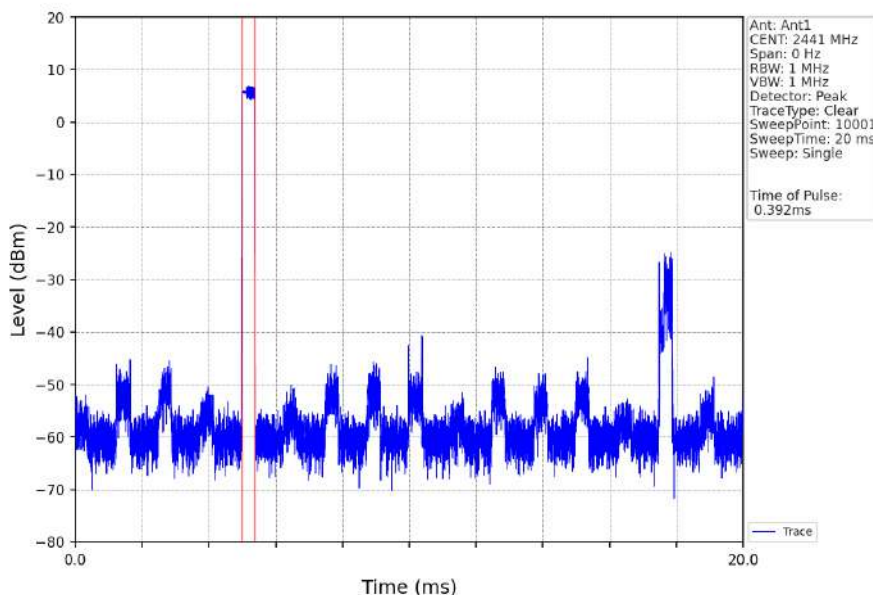
Pi/4DQPSK_2DH1_HOPP_Ant1_NTNV
