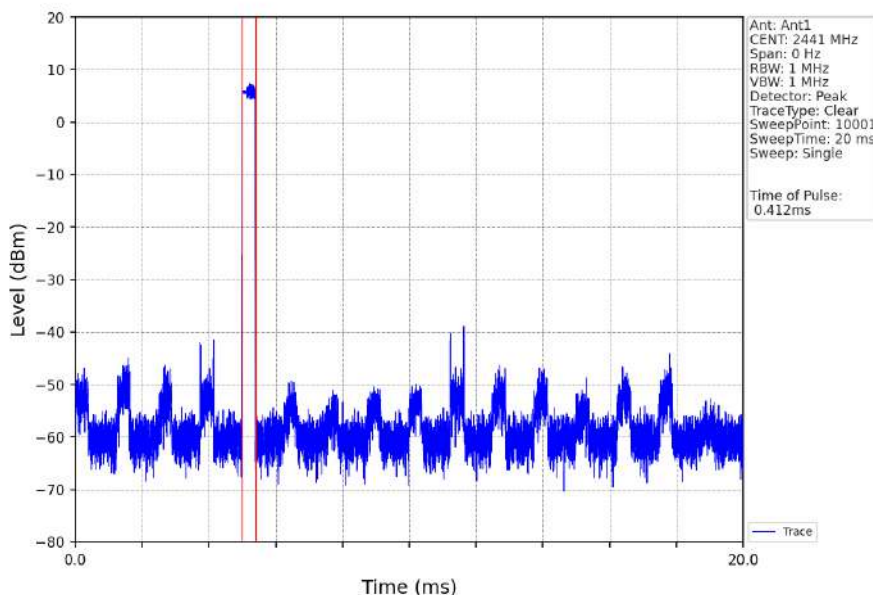
8DPSK_3DH1_HOPP_Ant1_NTNV
