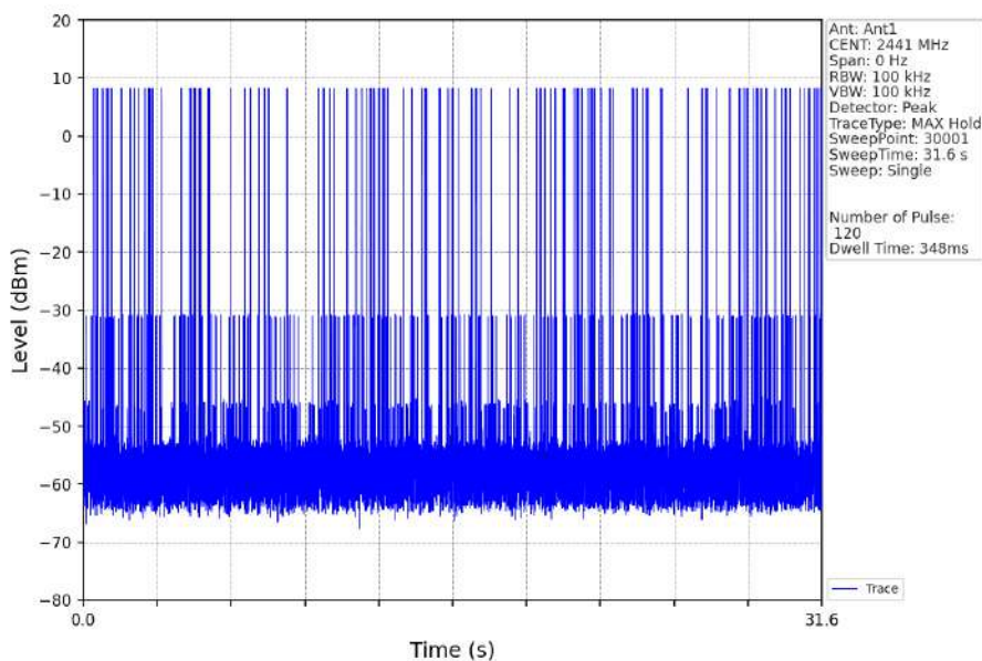
GFSK_DH5_HOPP_Ant1_NTNV
