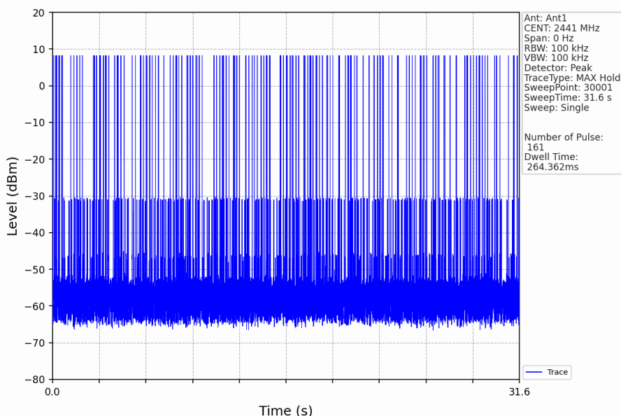
GFSK_DH3_HOPP_Ant1_NTNV
