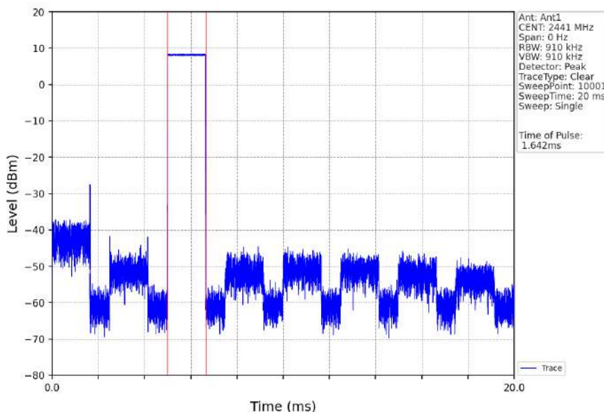
GFSK_DH3_HOPP_Ant1_NTNV
