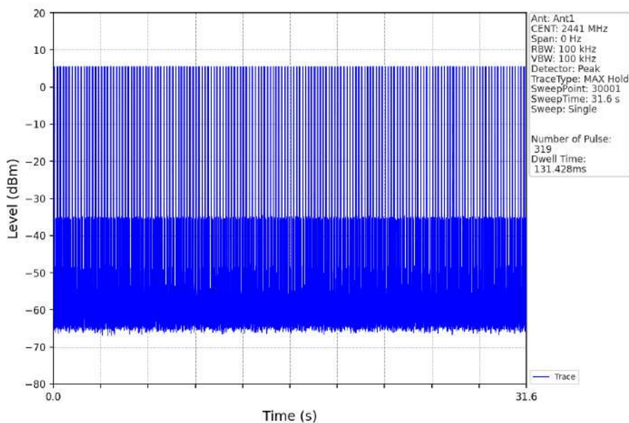
8DPSK_3DH1_HOPP_Ant1_NTNV
