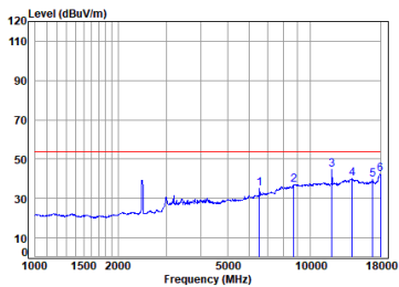
11n_40M_TX_CH_09_Vertical-Avg
