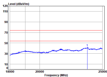
11n_40M_TX_CH_09_Horizontal
