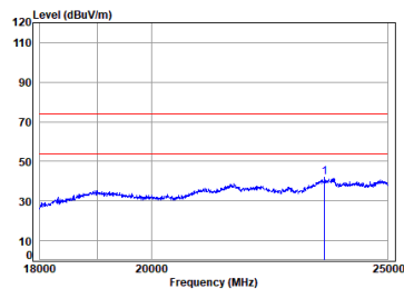
11n_40M_TX_CH_09_Vertical
