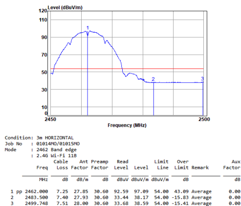
11b_TX_CH_11_Horizontal-Avg
