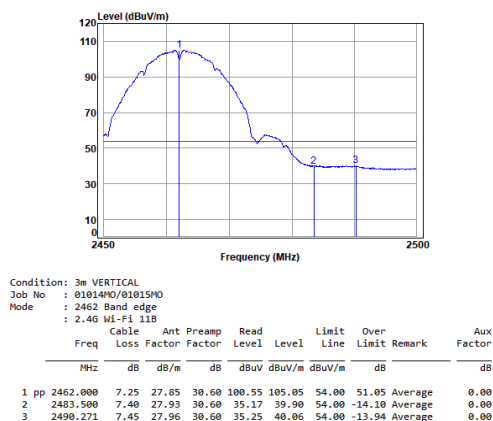
11b_TX_CH_11_Vertical-Avg
