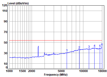
11n_40M_TX_CH_09_Horizontal-Avg
