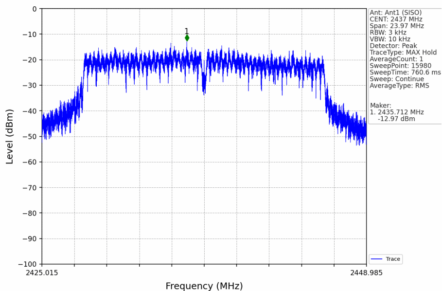
802.11n(HT20)_MCH_2437MHz_Ant1 (SISO)_NTNV
