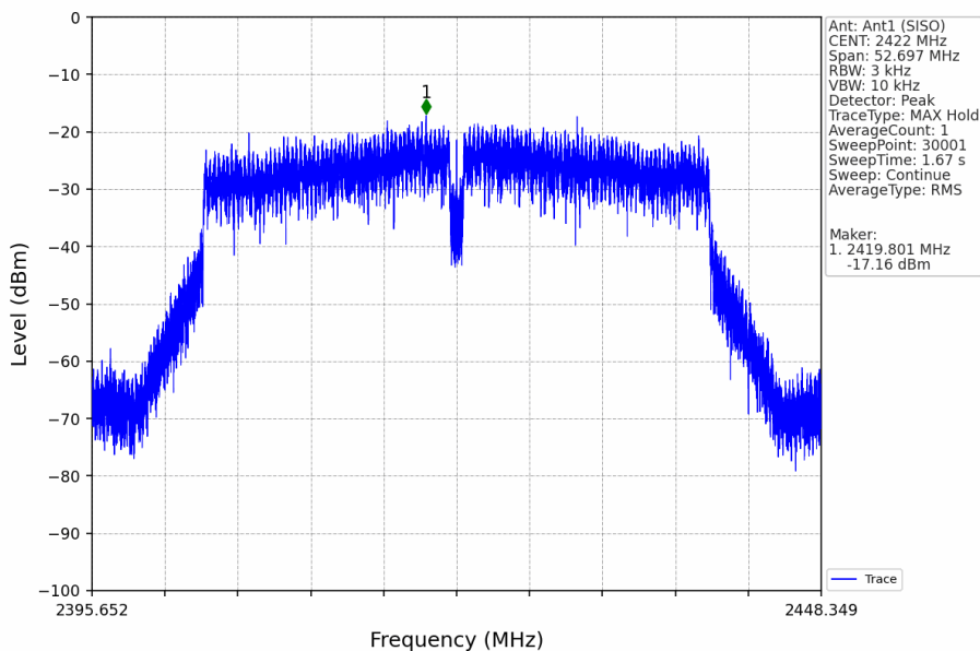
802.11n(HT40)_LCH_2422MHz_Ant1 (SISO)_NTNV
