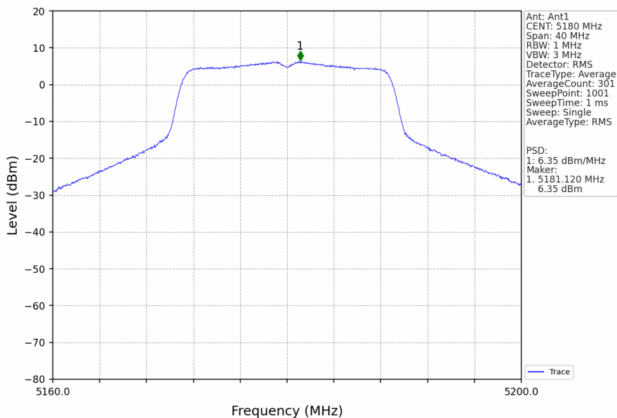
802.11n(HT20)_LCH_5180MHz_Ant1_NTNV
