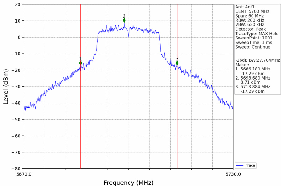
802.11n(HT20)_HCH_5700MHz_Ant1_NTNV
