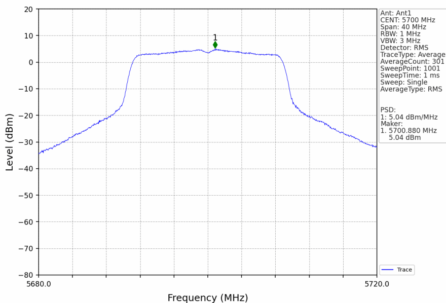
802.11n(HT20)_HCH_5700MHz_Ant1_NTNV
