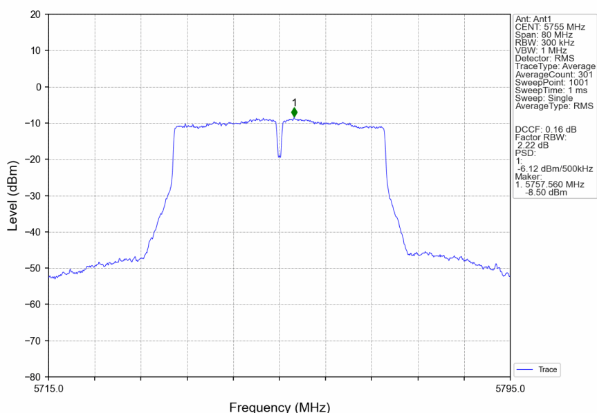
802.11ac(VHT40)_LCH_5755MHz_Ant1_NTNV
