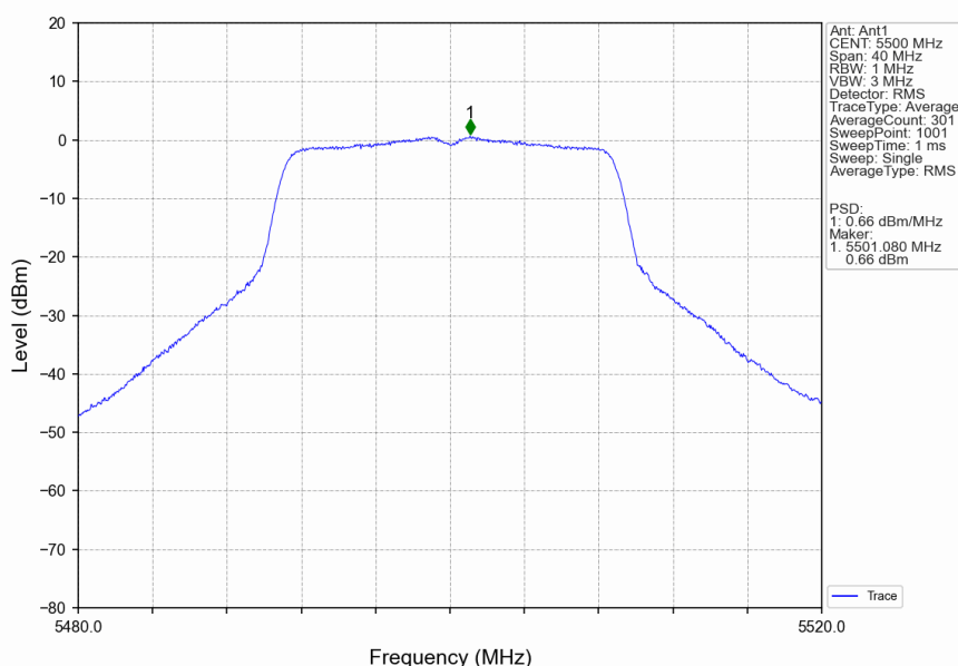
802.11ac(VHT20)_LCH_5500MHz_Ant1_NTNV
