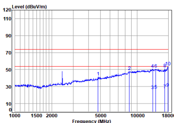
BT_DH5_TX_CH_39_Horizontal
