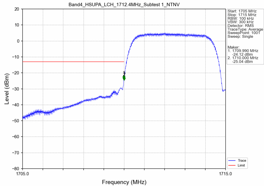
Band4_HSUPA_LCH_1712.4MHz_Subtest 1_NTNV
