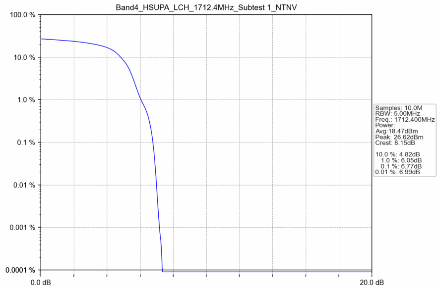
Band4_HSUPA_LCH_1712.4MHz_Subtest 1_NTNV
