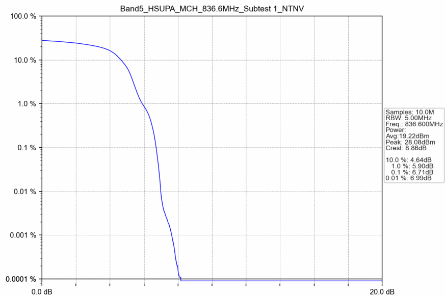
Band5_HSUPA_MCH_836.6MHz_Subtest 1_NTNV
