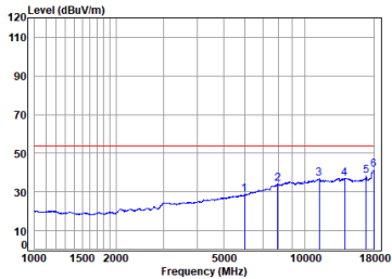
11n_40M_TX_CH_06_Vertical-Avg
