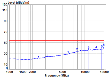
11n_40M_TX_CH_03_Horizontal-Avg
