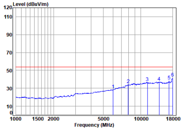
11n_40M_TX_CH_06_Horizontal-Avg
