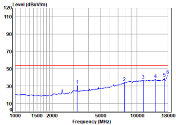
11n_40M_TX_CH_03_Vertical-Avg
