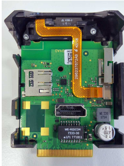
Photo 3: RF module up
