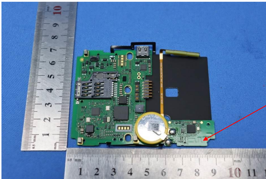
BLE antenna
