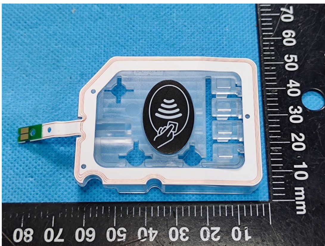
NFC Antenna
