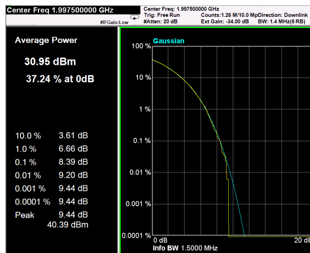
PAR measure example (LTE 1,4MHz QPSK)
