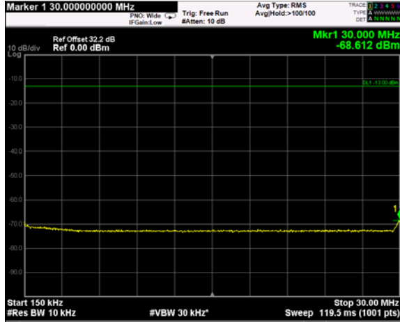
150kHz-30MHz
