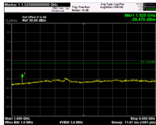
1GHz-8GHz
