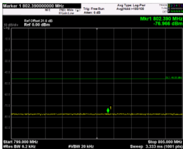
799MHz-805MHz
