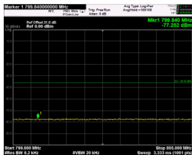
799MHz-805MHz
