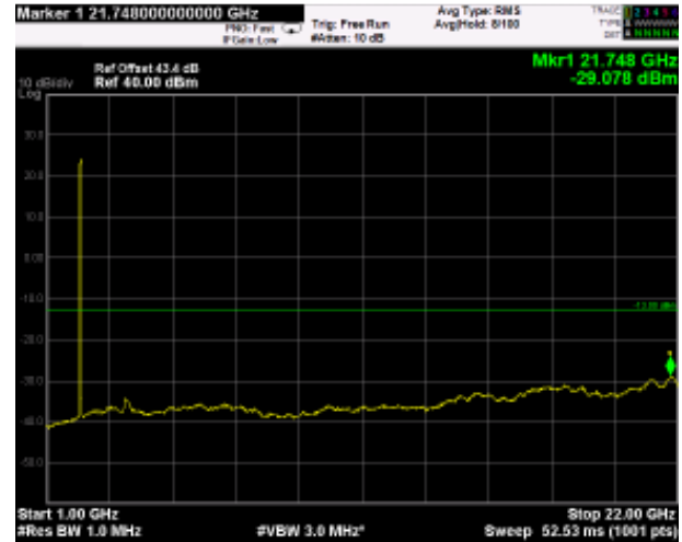
1GHz-22GHz
