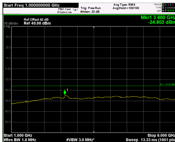
MSK SIGNAL, 1GHz-9GHz
