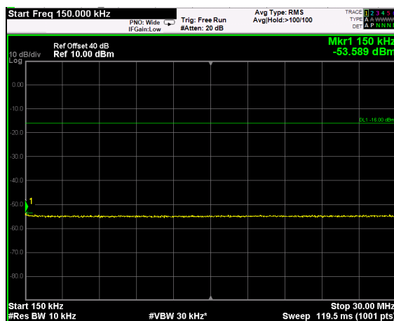
MSK SIGNAL, 150kHz-30MHz
