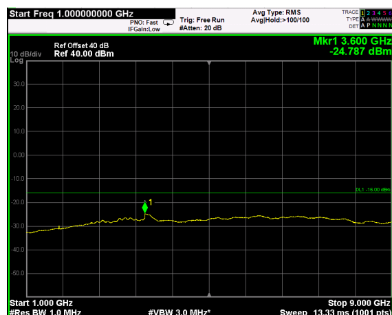
AWGN SIGNAL, 1GHz-9GHz
