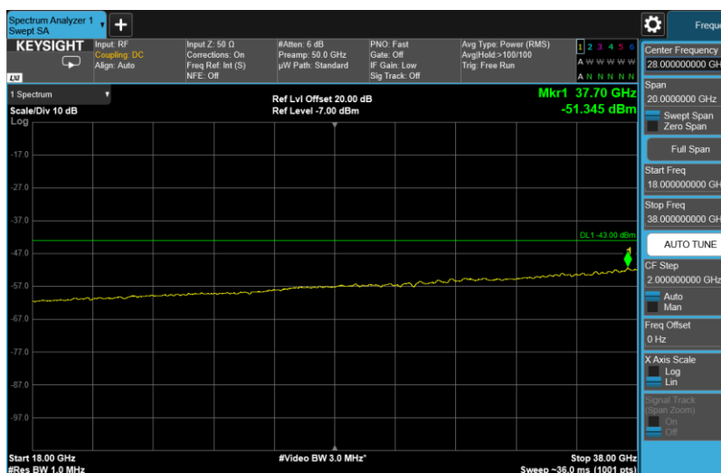
Channel: TOP, Modulation: QPSK, BW=15MHz, Range: 18GHz - 38GHz
