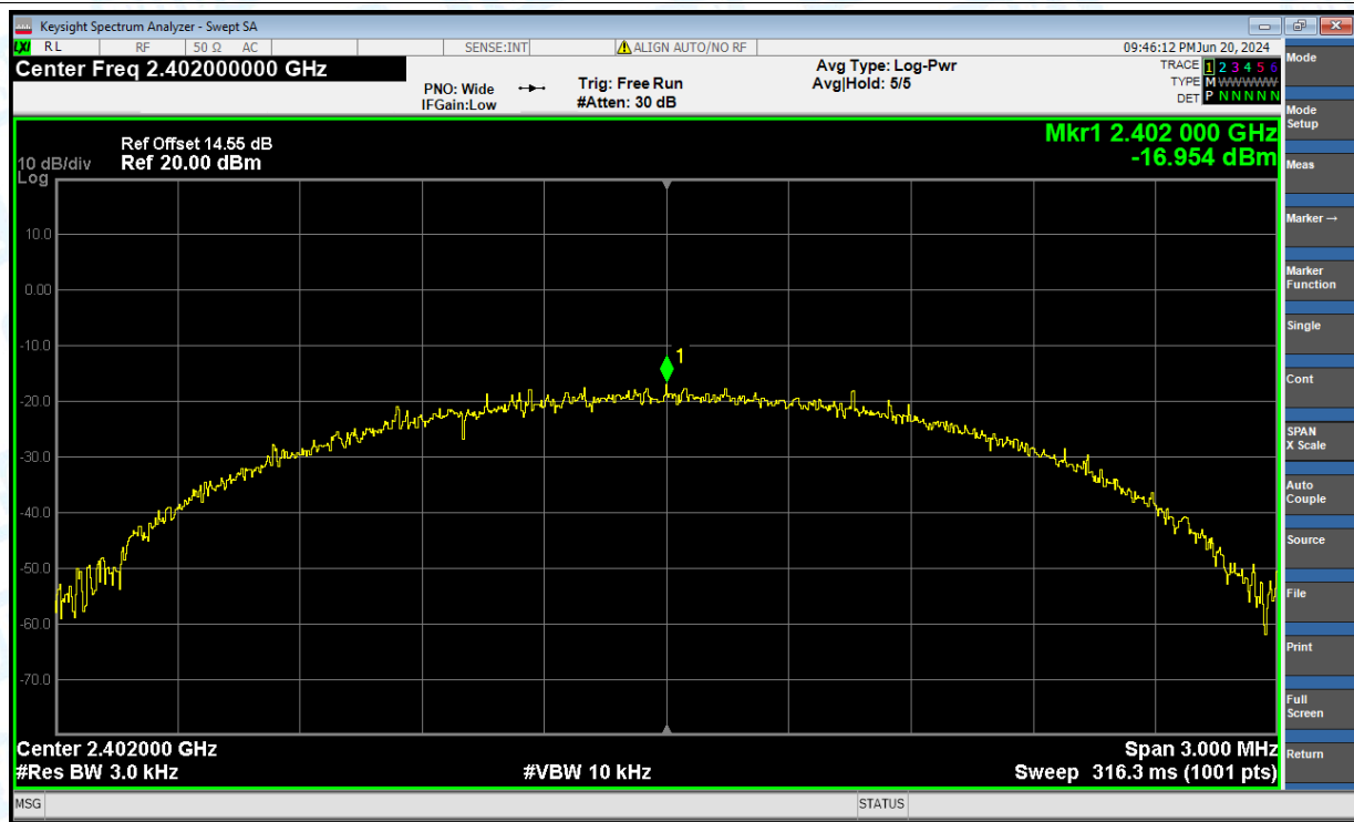
PSD NVNT BLE 2Mbps 2402MHz Ant1
