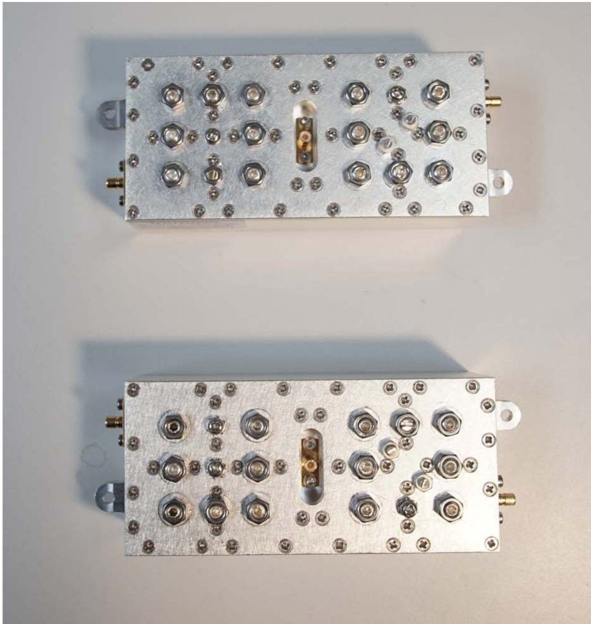
Duplexer 800MHz
