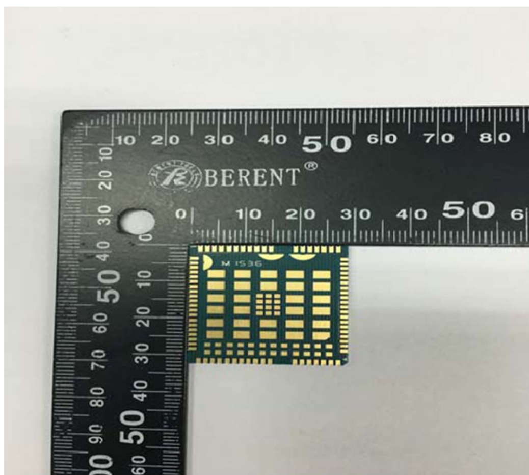
EUT -Rear Side
