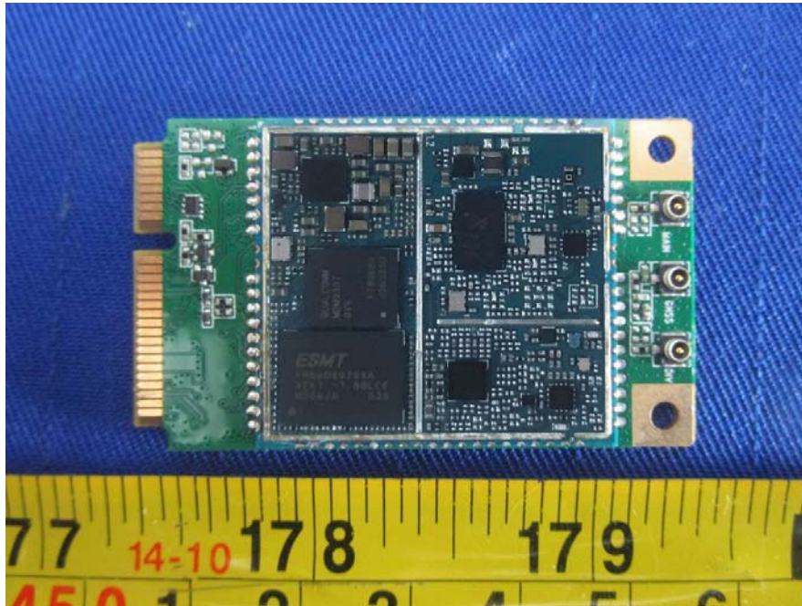
Model: EC25-V MiniPCIe , EC25-VD MiniPCIe EUT –Top View
