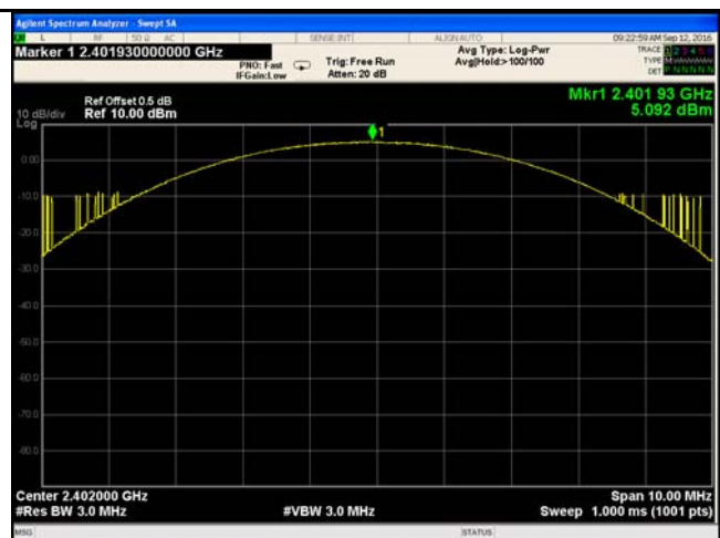
\pi/4 DQPSK Output power - Low CH 2402
