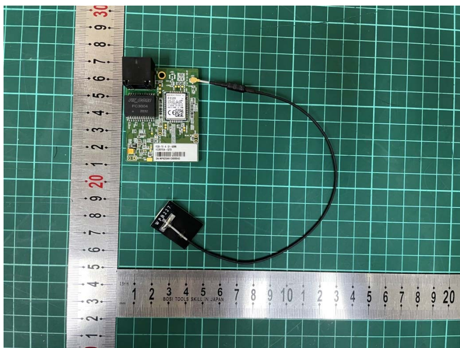
Antenna 3(45-2-000368)
