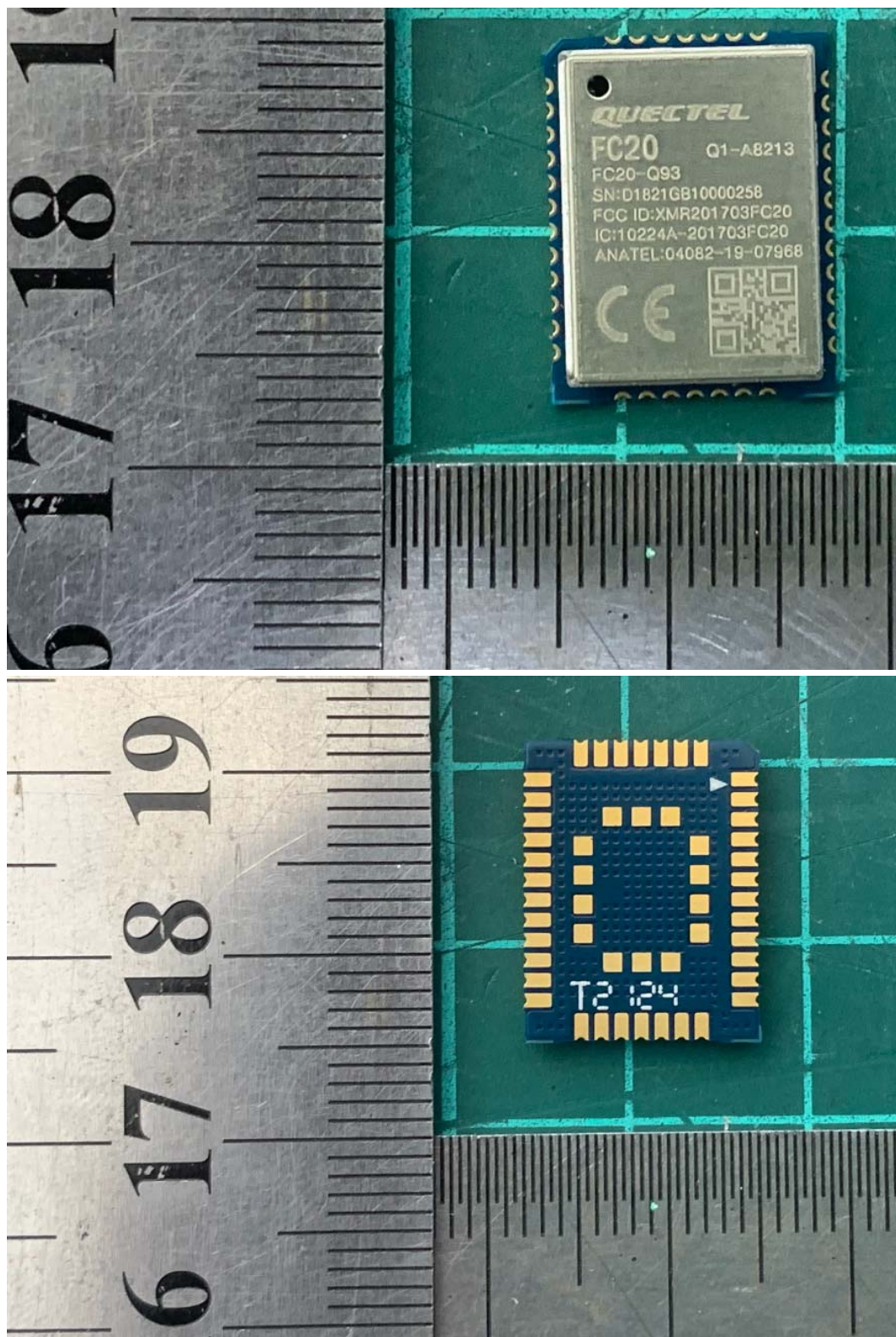
a: EUT
