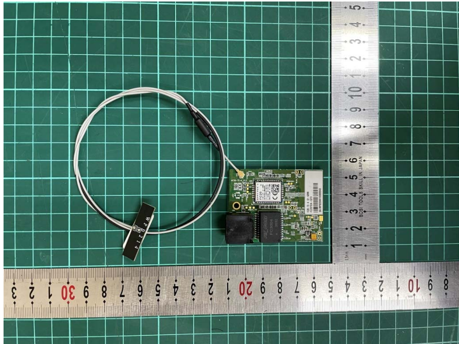
Antenna 4(45-2-000242)
