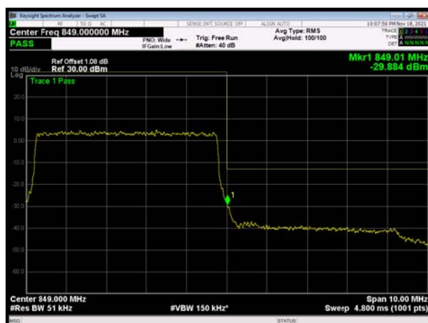
LTE Band 5 10MHz QPSK 1RB CH-High
